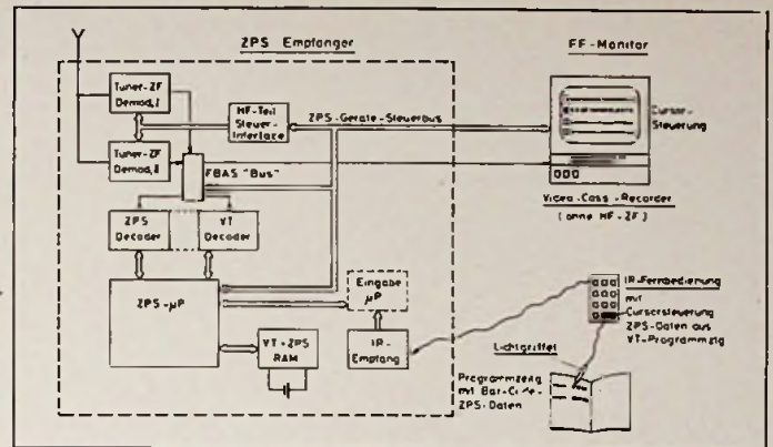
Bild 4. Prinzip eines Speicherfernsehers
