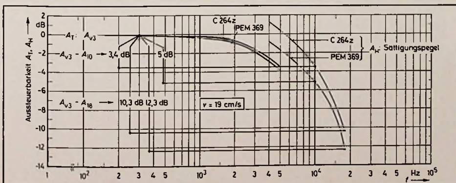
Bild 1. Aussteuerbarkeit des 1/4"-Referenzleerbandes C 264 z bei einer Bandgeschwindigkeit von 19 cm/s. Zum Vergleich die Kurven für die Bandsorte „PEM 369“ von Agfa, bezogen auf gleiche Tiefenaussteuerbarkeit
