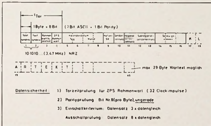
Bild 3. Codeaufbau einer ZPS-Datenzeile
