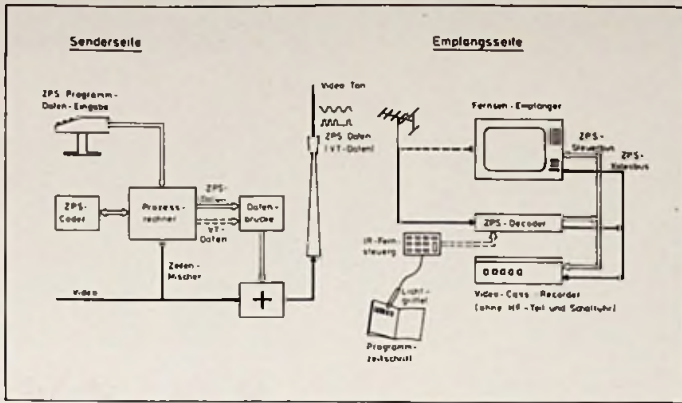
Bild 2. Prinzip des digitalen Kennungssystems „ZPS“
