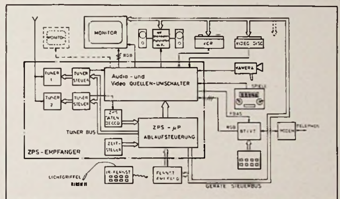
Bild 5. ZPS-gesteuertes Video-Komponenten-System
