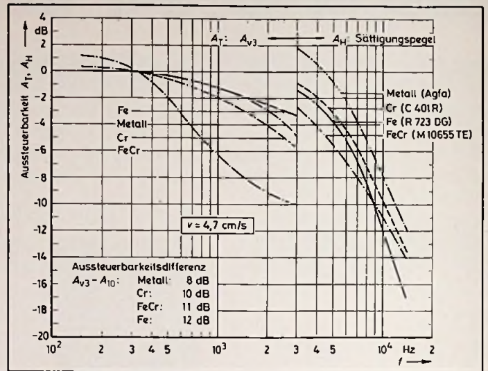
Bild 3. Aussteuerbarkeit von Cassetten-Referenzbändern ( v = 4,76 \text{ cm/s} ) bezogen auf gleiche Tiefenaussteuerung bei 333 Hz. Da das Referenzband für Metallbänder noch nicht festgelegt wurde, ist zum Vergleich das Metallband von Agfa in die Darstellung aufgenommen worden
