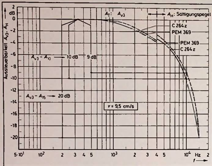
Bild 2. Aussteuerbarkeit des Referenzleerbandes C264 z und des Amateurbandes PEM369 bei der Bandgeschwindigkeit 9,5 cm/s bezogen auf gleiche Tiefenaussteuerbarkeit. Da die Aussteuerungsgrenze mit der aufgezeichneten Wellenlänge fällt, sind die Werte gegenüber Bild 1 schlechter
